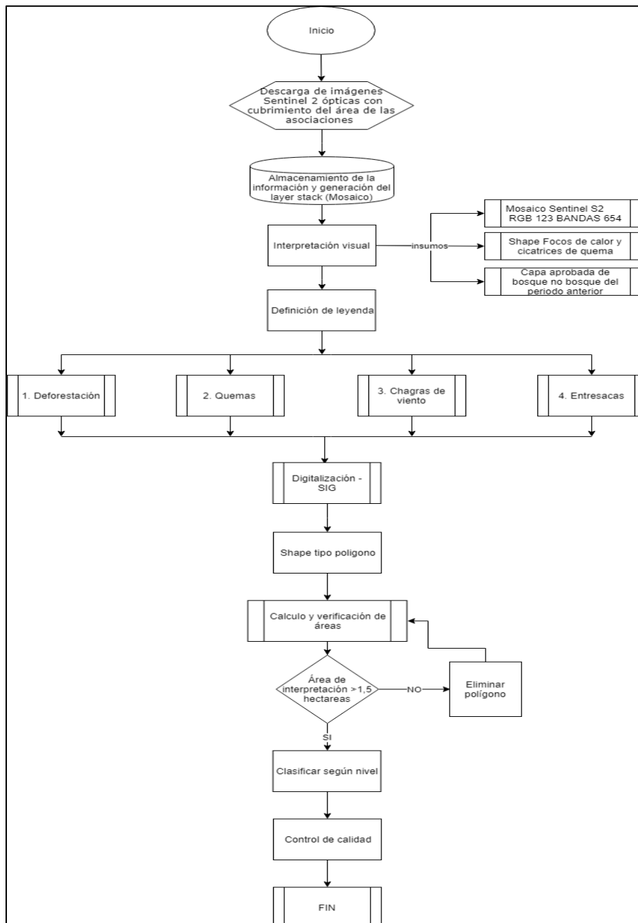
Figura 5 Diagrama de flujo de información para el seguimiento
